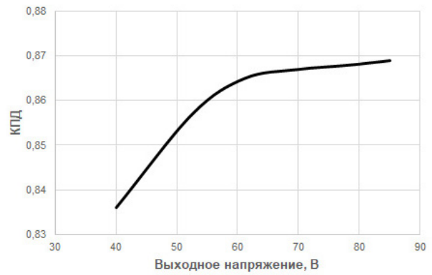
Рис. 2 - Зависимость КПД от выходного напряжения
